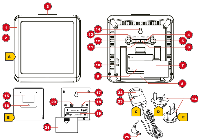
Fig. 1: Todas las piezas de la estación meteorológica (arriba), el sensor inalámbrico (abajo a la izquierda) y el adaptador de corriente con accesorios (abajo a la derecha).
