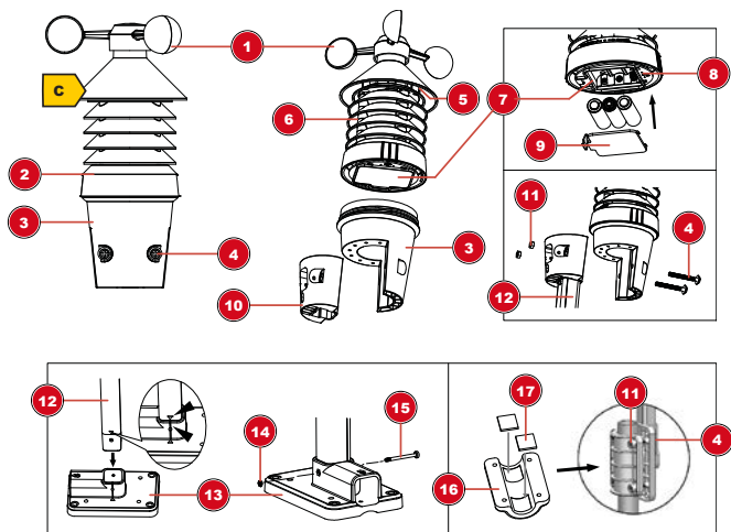
Fig. 2: Toutes les parties de la anémomètre
