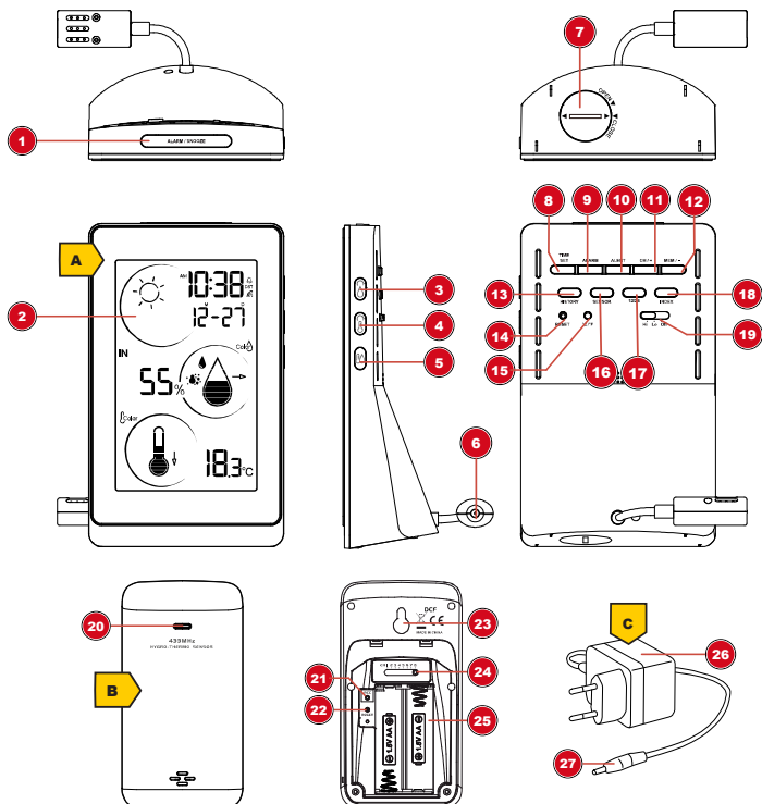
Abb. 1: Teileübersicht für Basisstation und Funksensor
