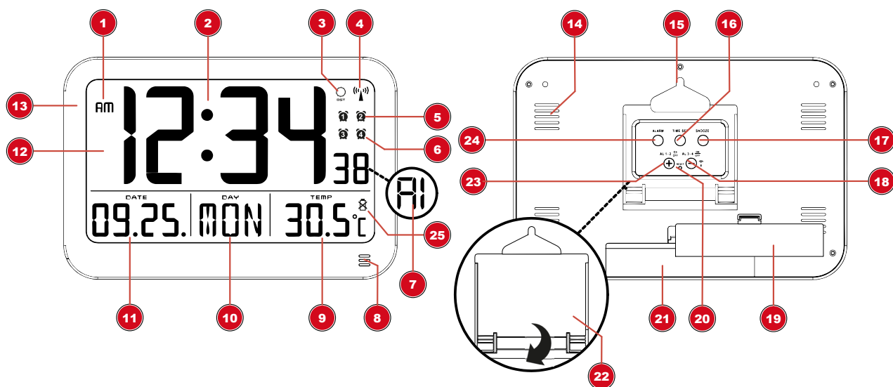
Fig. 1: Tutti i componenti dell'orologio da parete
