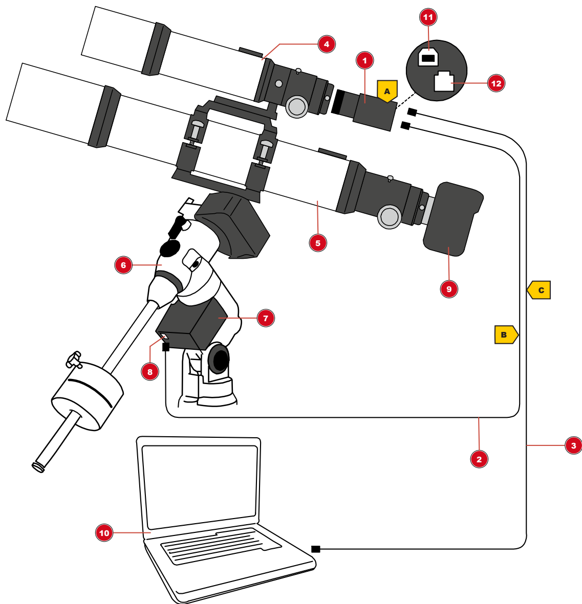
Fig. 1: Montaje de la cámara Full HD Deep-Sky como autoguía
